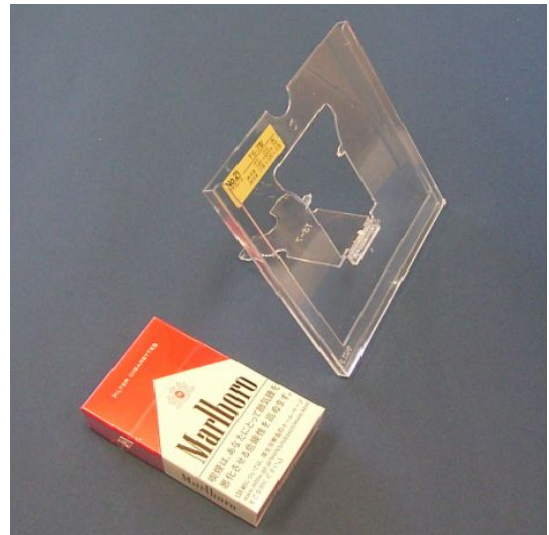
No.21 TS-7型 材質:スチロール 外寸 120 × 123.5 × 7 内寸 118 × 120 × 4
